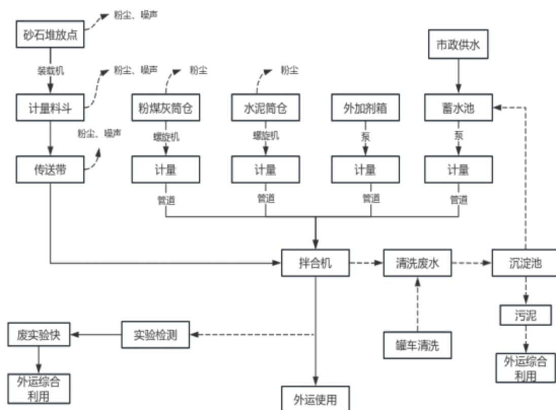
图 2-2 混凝土生产工艺流程图
