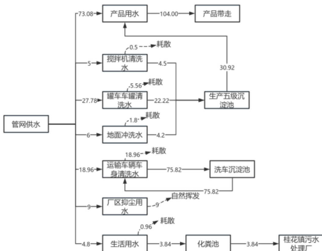
图 2-4 项目水平衡图 (单位: \text{m}^3/\text{d} )
